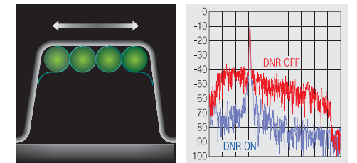
CONTOUR 特性概念図 デジタルノイズリダクション特性
