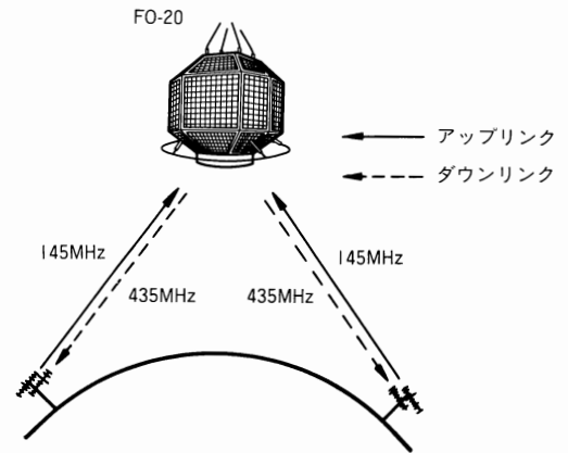
FO-20アナログ・モードの送受信周波数関係
