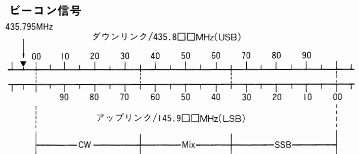
FO-20アナログ・モードの送受信周波数関係
