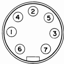
EXT CONT背面パネルから見た図
