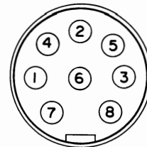
ACC4背面パネルから見た図
